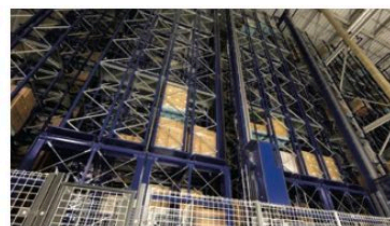
自動倉庫
